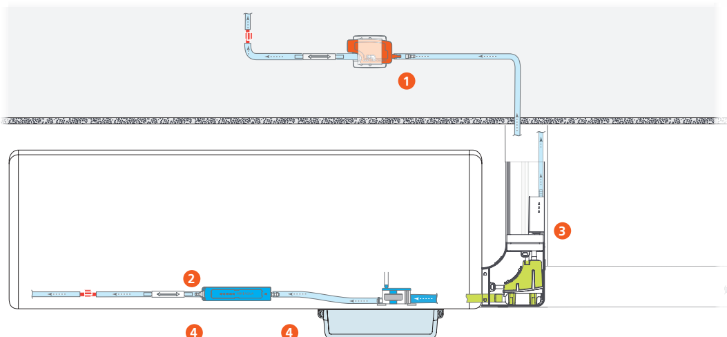
1 W podwieszanym suficie (uwaga: w zestawie uchwyt tłumiący wibracje) 2 Wewnątrz klimatyzatora 3 W corytce 4 Pod klimatyzatorem
